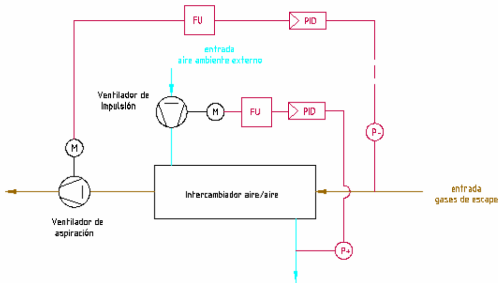
Figura 4. Sistema de regulación del funcionamiento de los ventiladores de impulsión y de aspiración en el intercambiador aire/aire.
