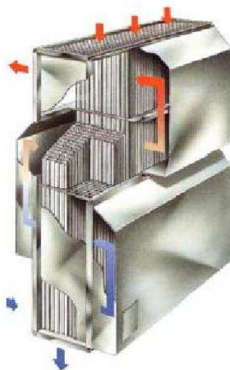
Figura 1. Modelo del intercambiador de tubos y carcasa.
