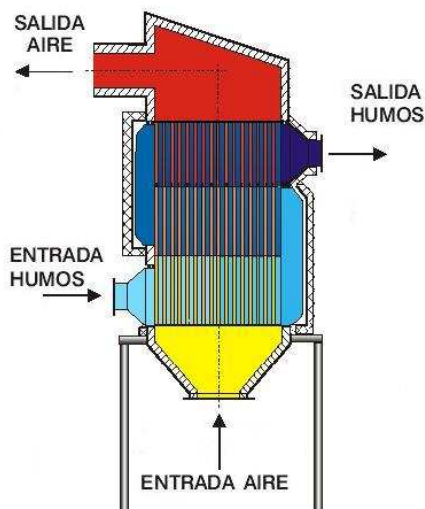
Figura 2. Sentidos de circulación del flujo de aire exterior y del flujo de gases de escape.
