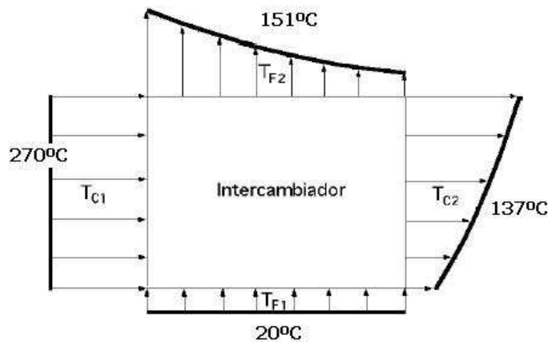
Figura 5. Evolución de las temperaturas del flujo caliente y del frío a la entrada/salida del intercambiador.
