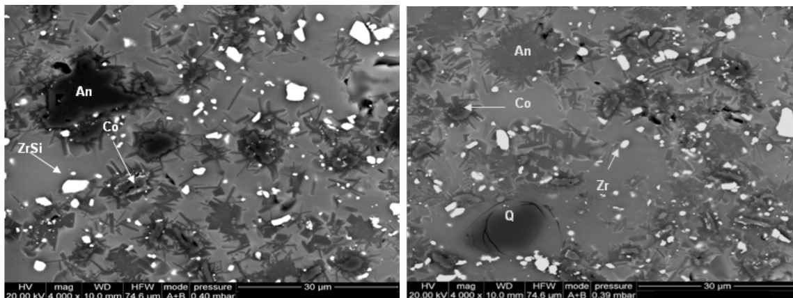
Figura 5 Sección transversal del vidriado PG. Estructuras cristalinas identificadas: ZrSi= Circón ( \text{ZrSiO}_4 ), Co= Corindón ( \text{Al}_2\text{O}_3 ), Geh= Gehlenita( \text{Ca}_2\text{Al}_2\text{SiO}_7 ) y Gah= Gahnita ( \text{ZnAl}_2\text{O}_4 ) (4000x) (20kV)
