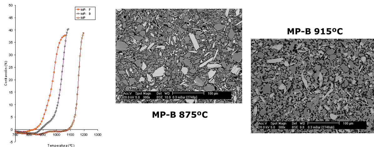
Figura 2 Curva de contracción de los esmaltes MP, MP-B y MP-F y las micrografías del esmalte preparado con materias primas y la nueva materia prima de boro durante los primeros estadios de la sinterización.
