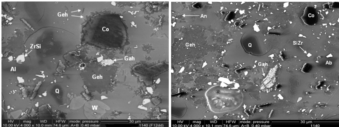
Figura 4 Sección transversal del vidriado EMG-F y EMG-V. Estructuras cristalinas identificadas: Q= Cuarzo ( \text{SiO}_2 ), Co= Corindón ( \text{Al}_2\text{O}_3 ), ZrSi= Circón ( \text{ZrSiO}_4 ) y Geh= Gehlenita( \text{Ca}_2\text{Al}_2\text{SiO}_7 ) (10 kV) (4000x)
