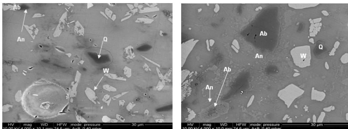
Figura 3 Sección transversal del vidriado EMA-F y EMA-B. Estructuras cristalinas identificadas: Q= Cuarzo ( \text{SiO}_2 ), W= Wollastonita ( \text{CaSiO}_3 ), An=Anortita ( \text{CaAl}_2\text{Si}_2\text{O}_8 ) y Ab= Albita ( \text{NaAlSi}_3\text{O}_8 )
