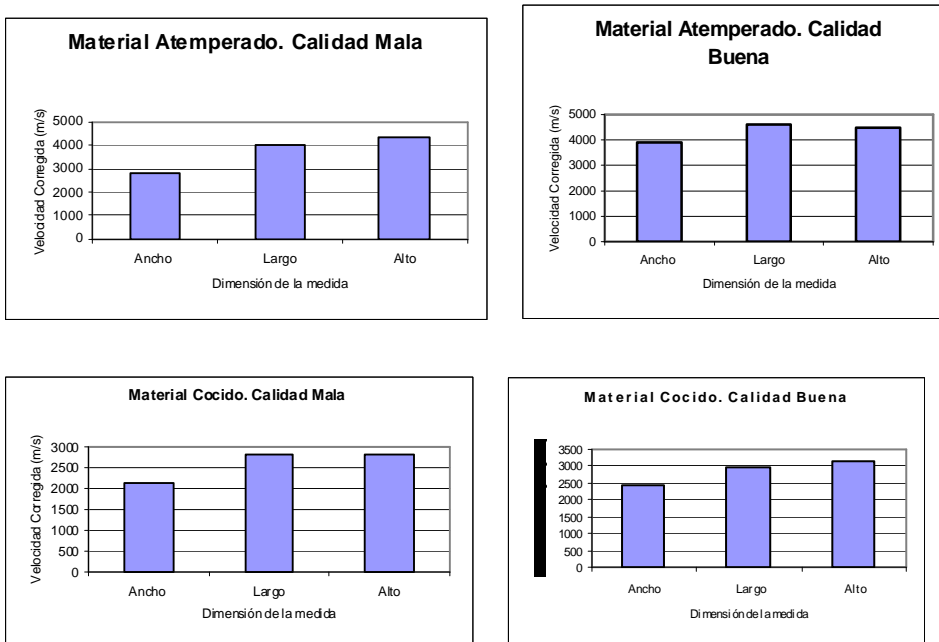
Grafica 1.- Velocidades corregidas de los dos materiales y las dos calidades en las tres dimensiones (5).
