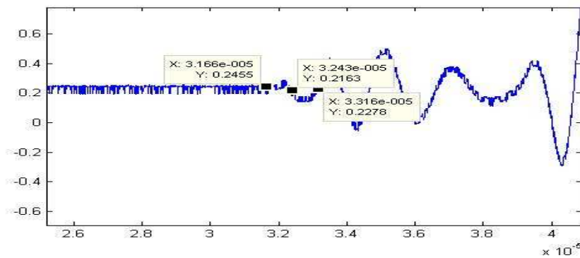
Figura 1.- Señal de ultrasonidos con los valores t_0 , t_1 y t_2 (1).
